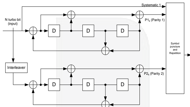
Gambar 3. Struktur turbo encoder dengan \frac{1}{3} diadaptasi dari [3]
