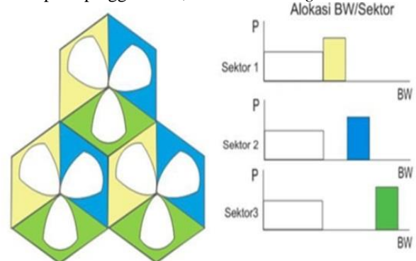
Gambar 3.1 Alokasi Power dan Frekuensi pada FFR
