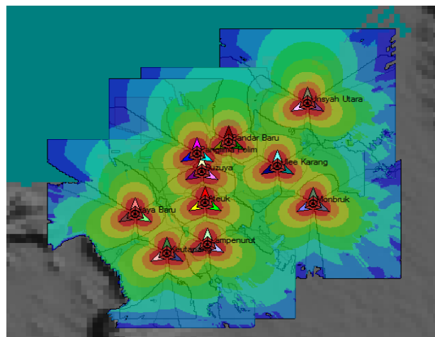
Gambar 4.2 Hasil Simulasi LTE FFR
